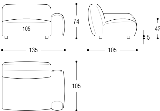
Element cm 135 right
