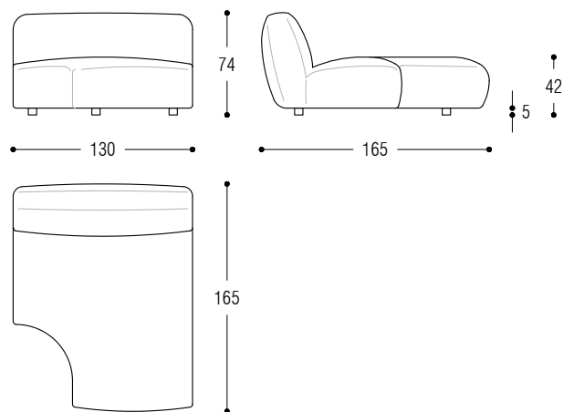
Endunit cm 165 right
